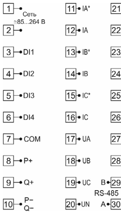
Рис. 4 – Схема подключения P99-MZ-3-0.5-RS485
