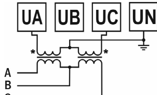
Рис. 10 – Подключение трансформатора напряжения x/380 В (трехфазная цепь без нейтрали)
