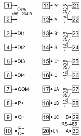
Рис. 6 – Схема подключения P99-MZ-3-0.5-4K-RS485
