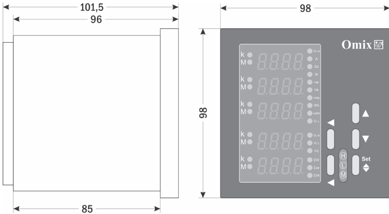
Рис. 3 – Размеры прибора
