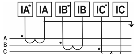
Рис. 12 – Подключение трансформатора тока x/5 А
