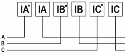
Рис. 11 – Подключение тока напрямую до 5 А
