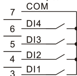
Рис. 13 – Схема подключения импульсных выходов
