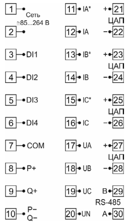
Рис. 5 – Схема подключения P99-MZ-3-0.5-4I420-RS485
